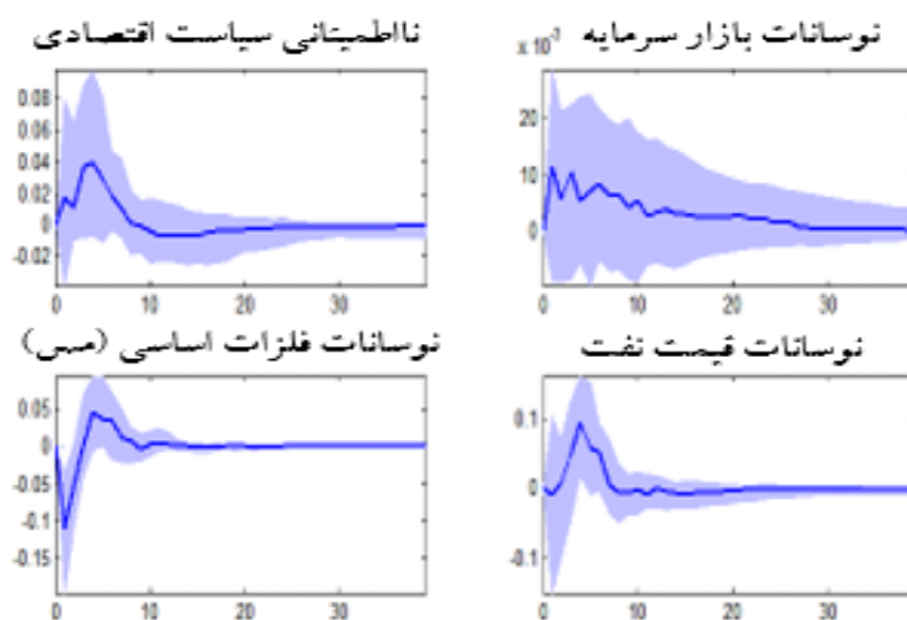
نمودار ۲. واکنش متغیرهای تحقیق به شوک وارد شده از ناحیه ناطمینانی سیاست‌های اقتصادی
