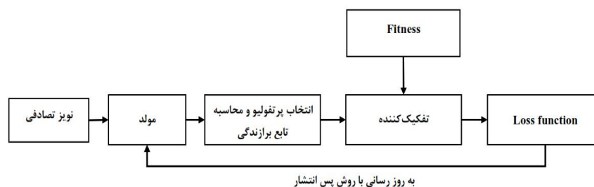
شکل ۳. شماتیک شبکه GAN.
