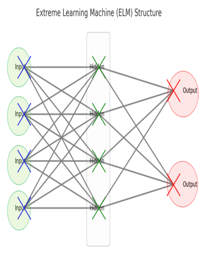
شکل ۴. ساختار مدل ELM.
