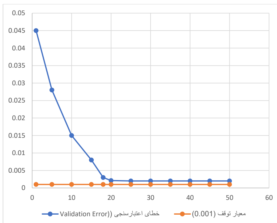
شکل ۸. بهینه‌سازی GWO - خطا در طول تکرارها. منبع: نگارندگان
