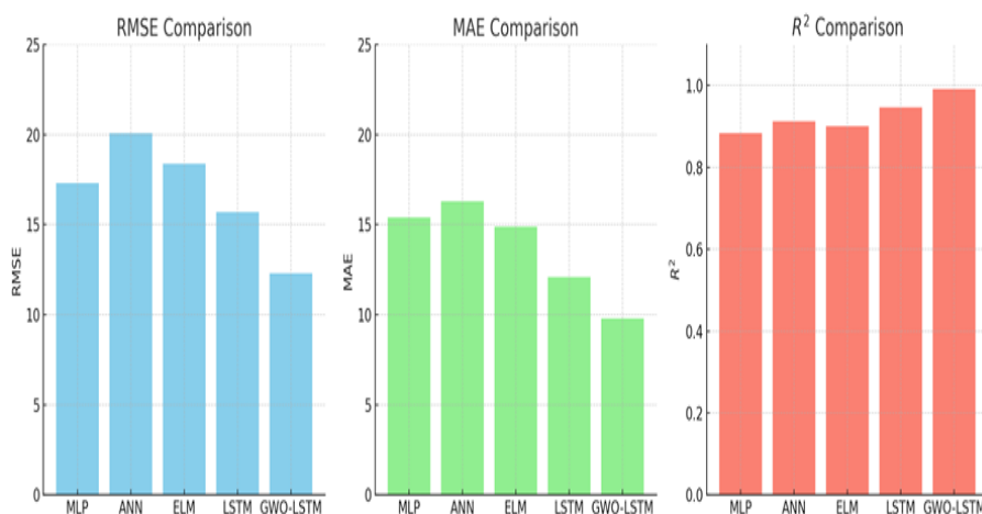
شکل ۹. مقایسه عملکرد روش‌ها.
