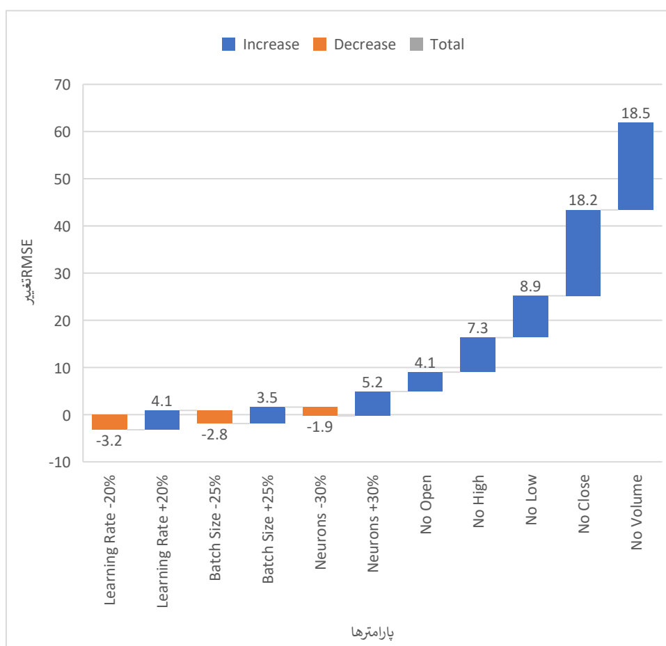
شکل ۷. نمودار حساسیت مدل GWO-LSTM
