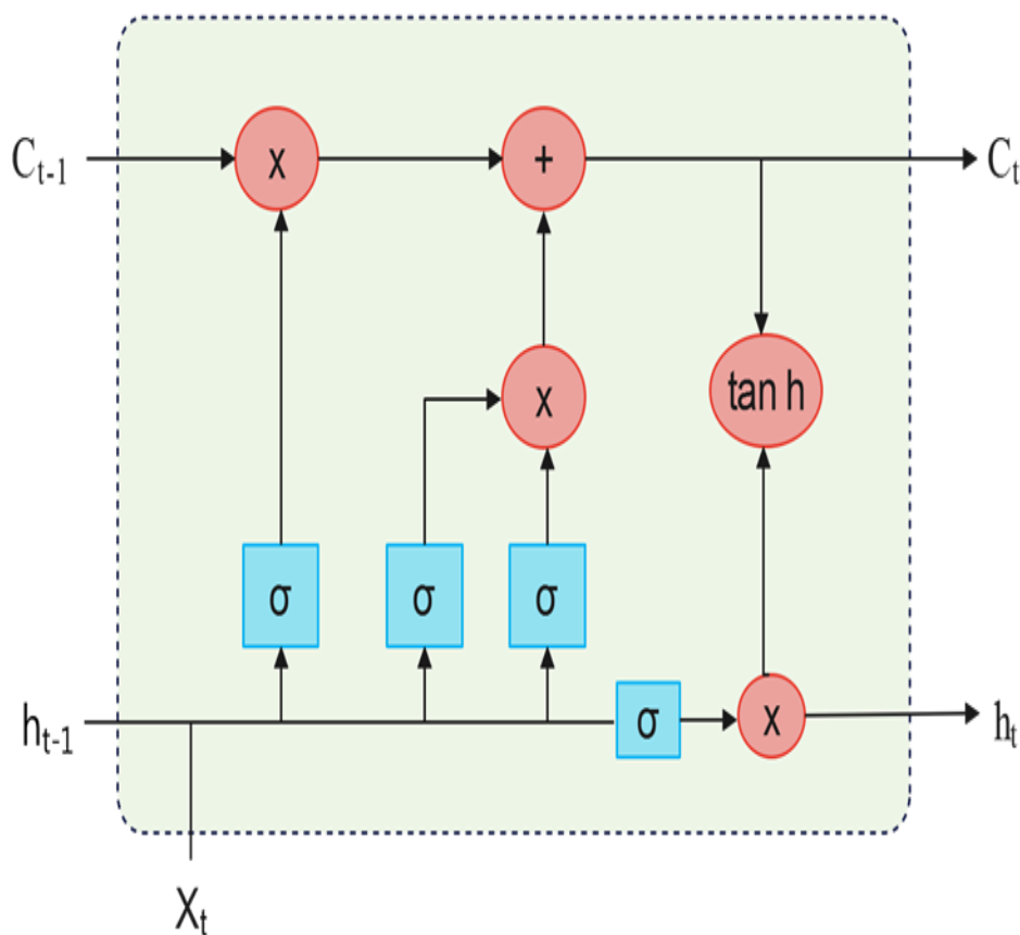
شکل ۱. ساختار مدل LSTM.
