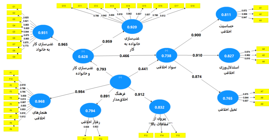
شکل ۲- مدل ساختاری در حالت تخمین ضرایب استاندارد
