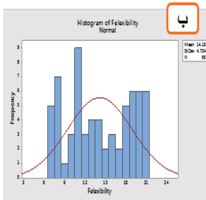
شکل ۲. الف) نمودار هیستوگرام برای متغیر ریسک، ب) نمودار هیستوگرام برای متغیر انعطاف‌پذیری، ج) نمودار هیستوگرام برای متغیر شریعت مأخذ: یافته‌های پژوهش
