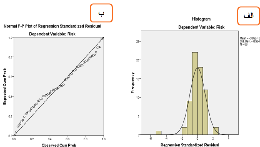
شکل ۱. الف) نمودار هیستوگرام باقیمانده مدل رگرسیون ساخته شده؛ ب) نمودار برازش باقیمانده استاندارد متغیر ریسک
