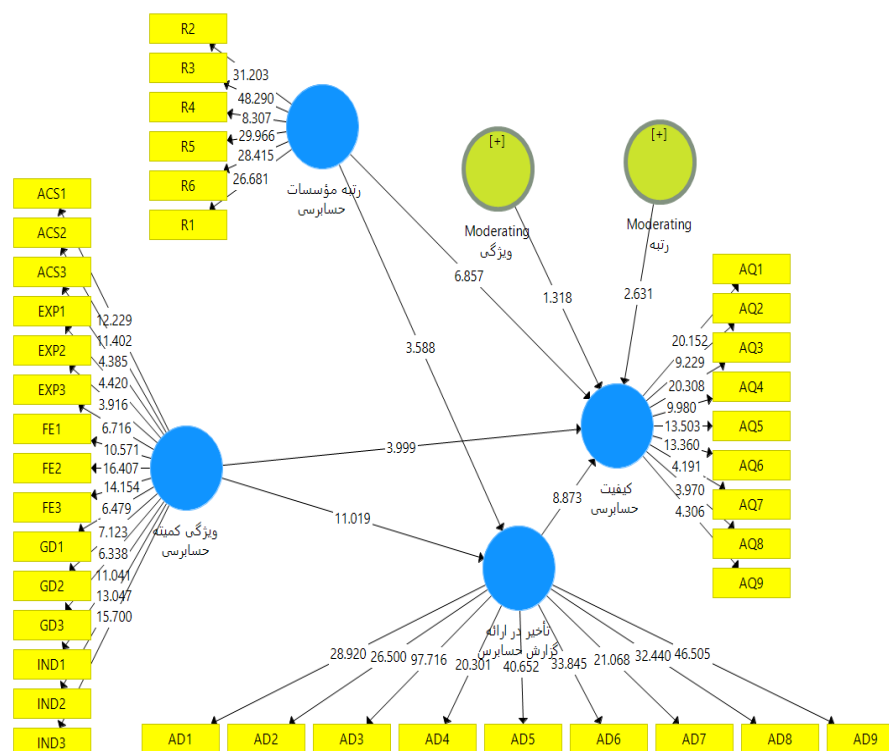
شکل ۳: بوت استرپ (مقادیر t)
