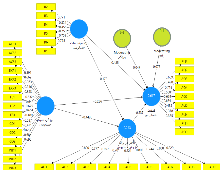
شکل ۲: مدل برازش شده در حالت تخمین استاندارد
