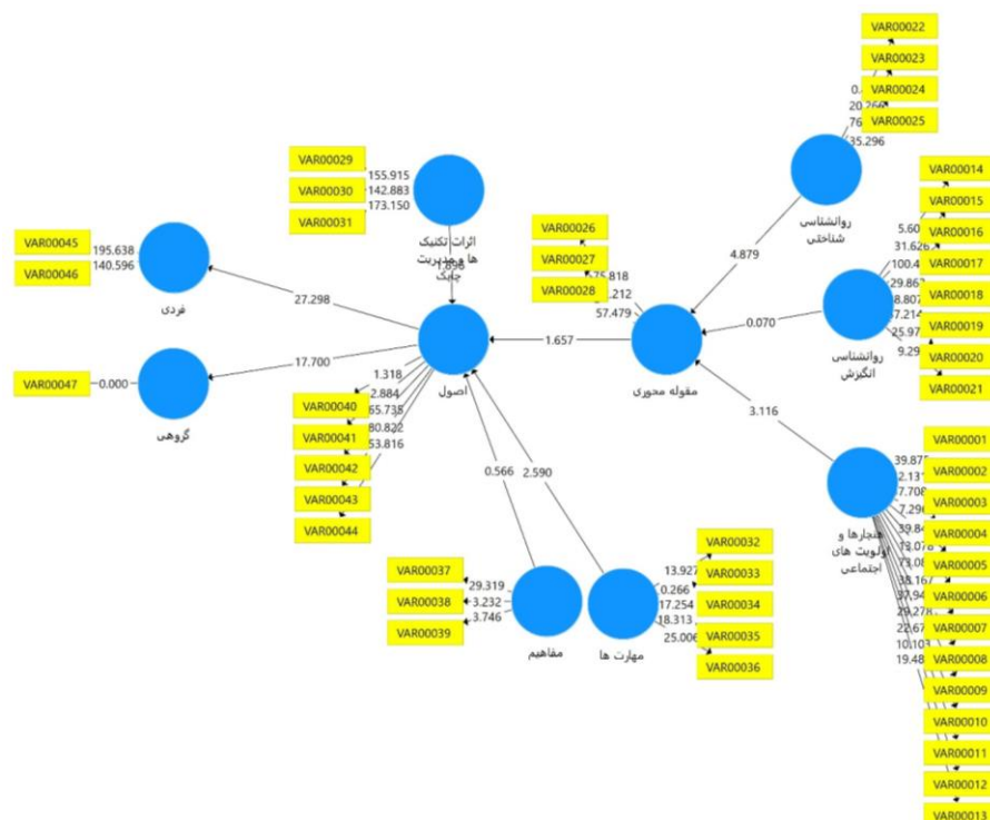
نمودار ۲: مدل اندازه گیری در حالت معنادار کلی
